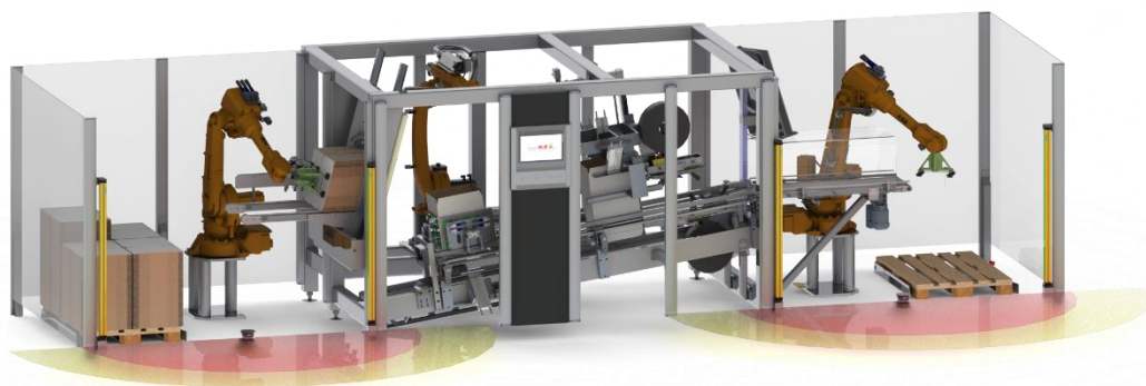
Bild 1 - Robot-Flexline: höchste Flexibilität auf engstem Raum
